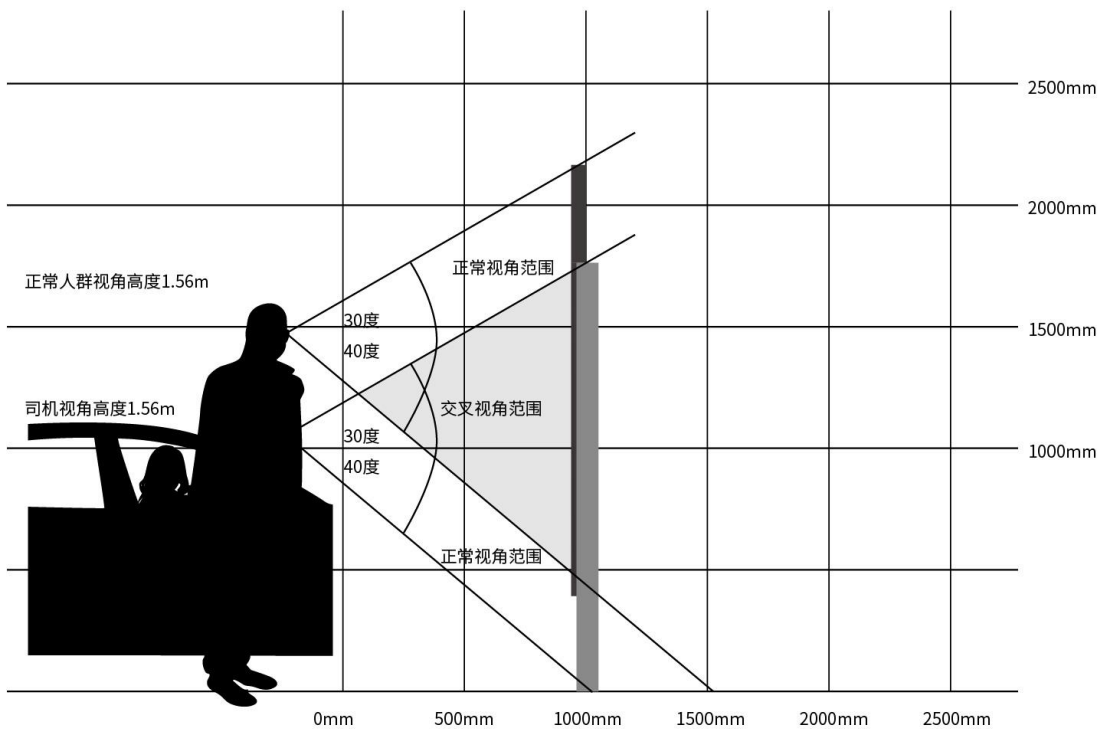
近距离观看导向标示时，标识设置最佳高度确定方法
